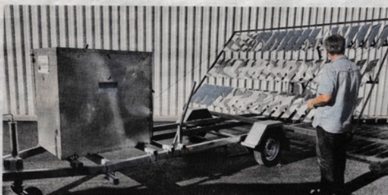
Le four solaire a été présenté devant les locaux de la Biocoop de Louviers. ©La Dépêche de Louviers
